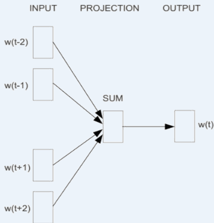
CBOW
